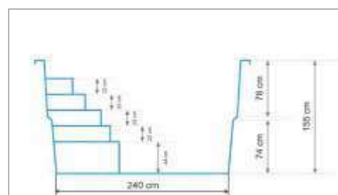
RZUT Z BOKU 300x155 cm
