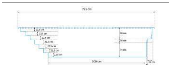
RZUT Z BOKU 725x155 cm
