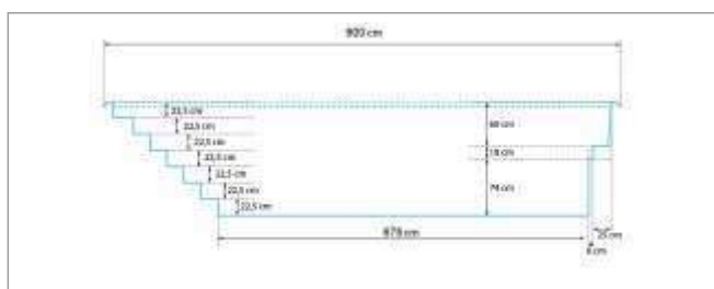
RZUT Z BOKU
