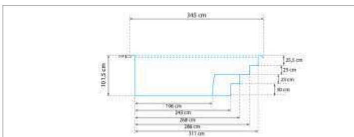
RZUT Z BOKU 345x101,5 cm
