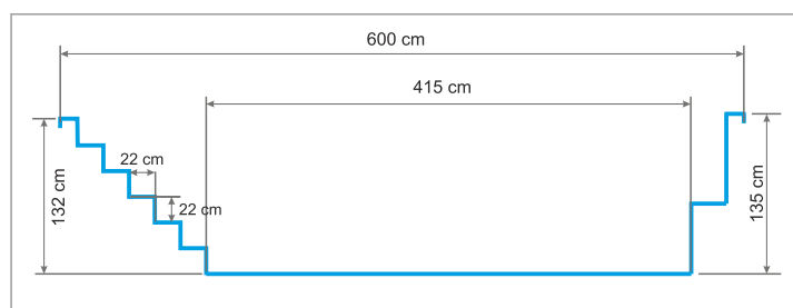
RZUT Z BOKU 600x135 cm
