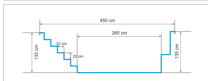
RZUT Z BOKU 450x135 cm
